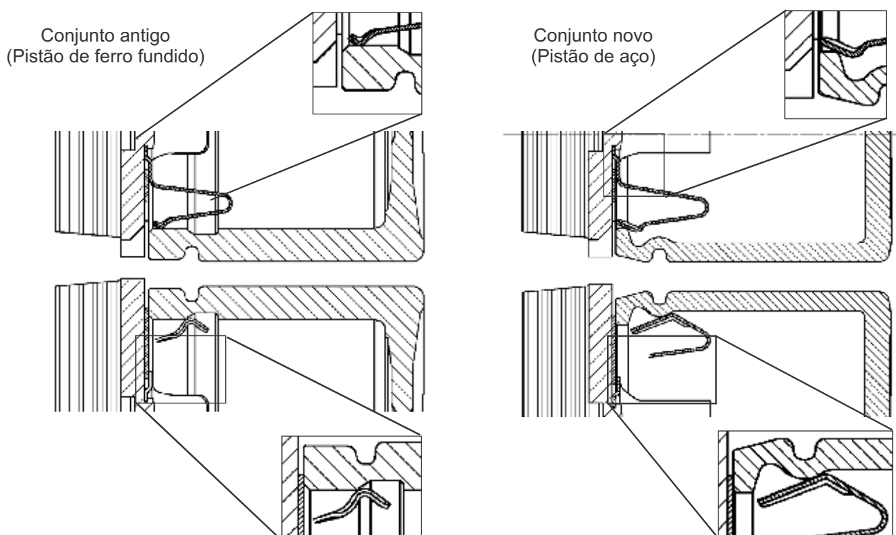
Perfil da mola da pastilha para Pistão de Ferro Fundido
