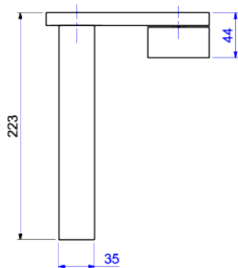
Desenho Técnico
