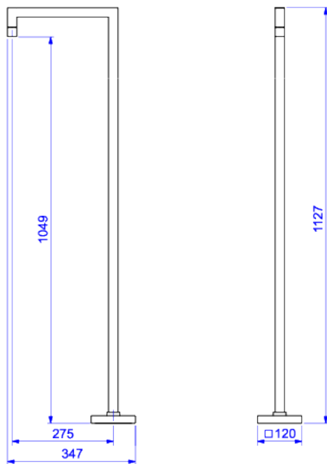
Desenho Técnico
