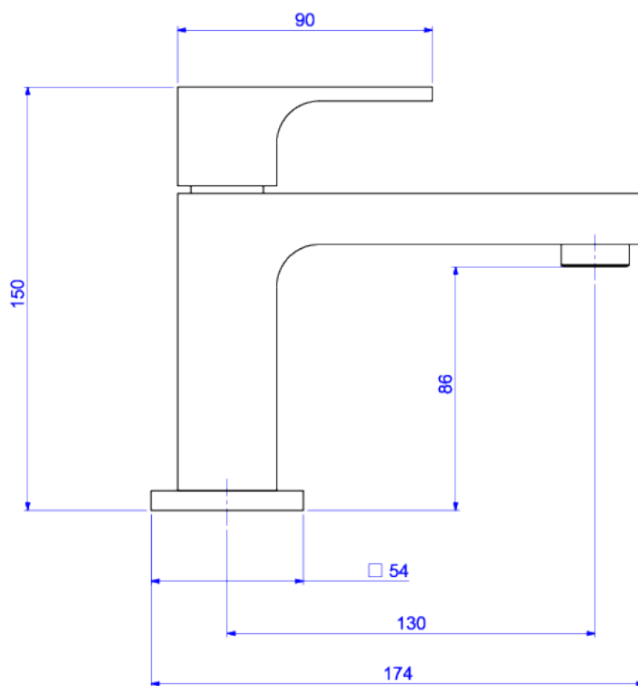
Desenho Técnico
