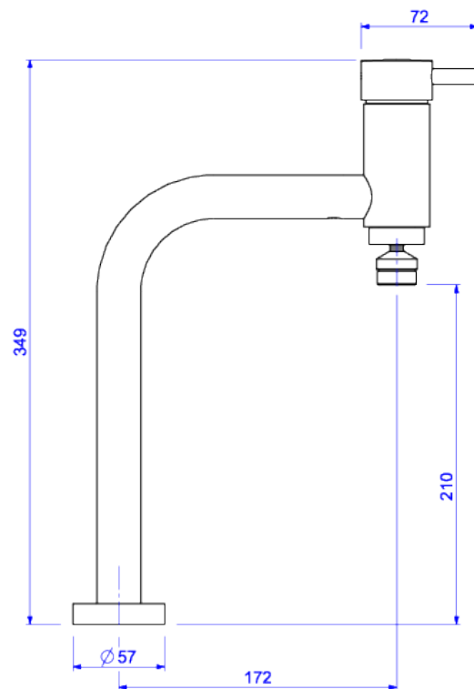
Desenho Técnico
