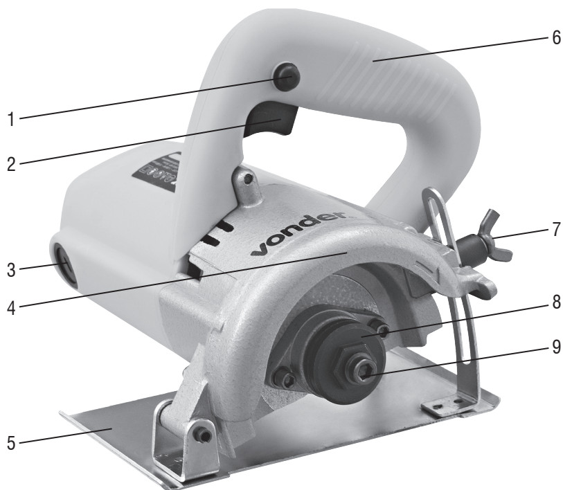
Fig. 1 – Componentes da ferramenta
